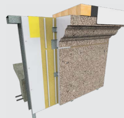
Parapet Cornice
