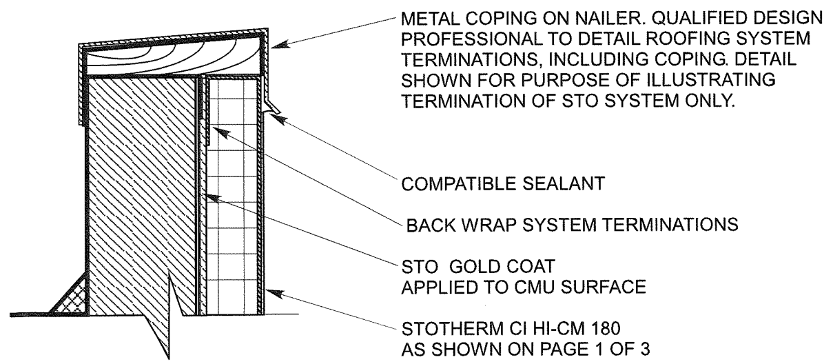
PARAPET CAP
