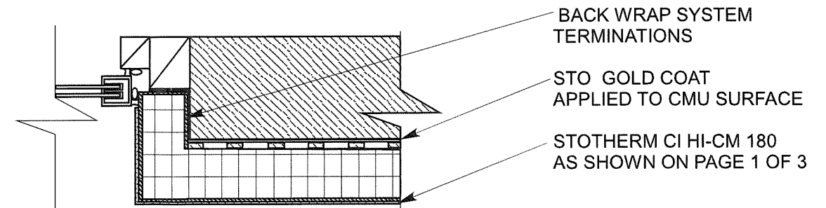
WINDOW JAMB
