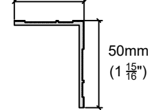
StoVentro L-Profile
